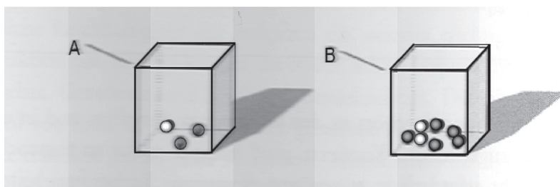
3. ábra. PISA-feladat
